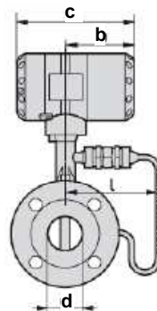
Вид спереди
