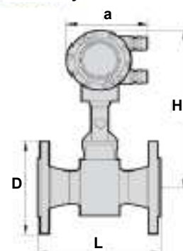
Вид сбоку
