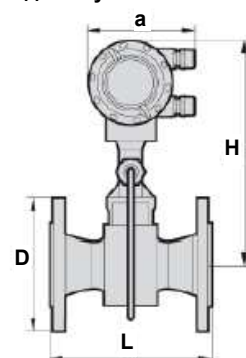
Вид сбоку
