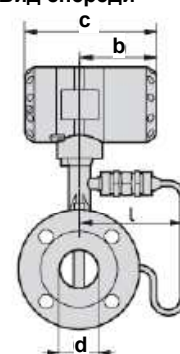
Вид спереди
