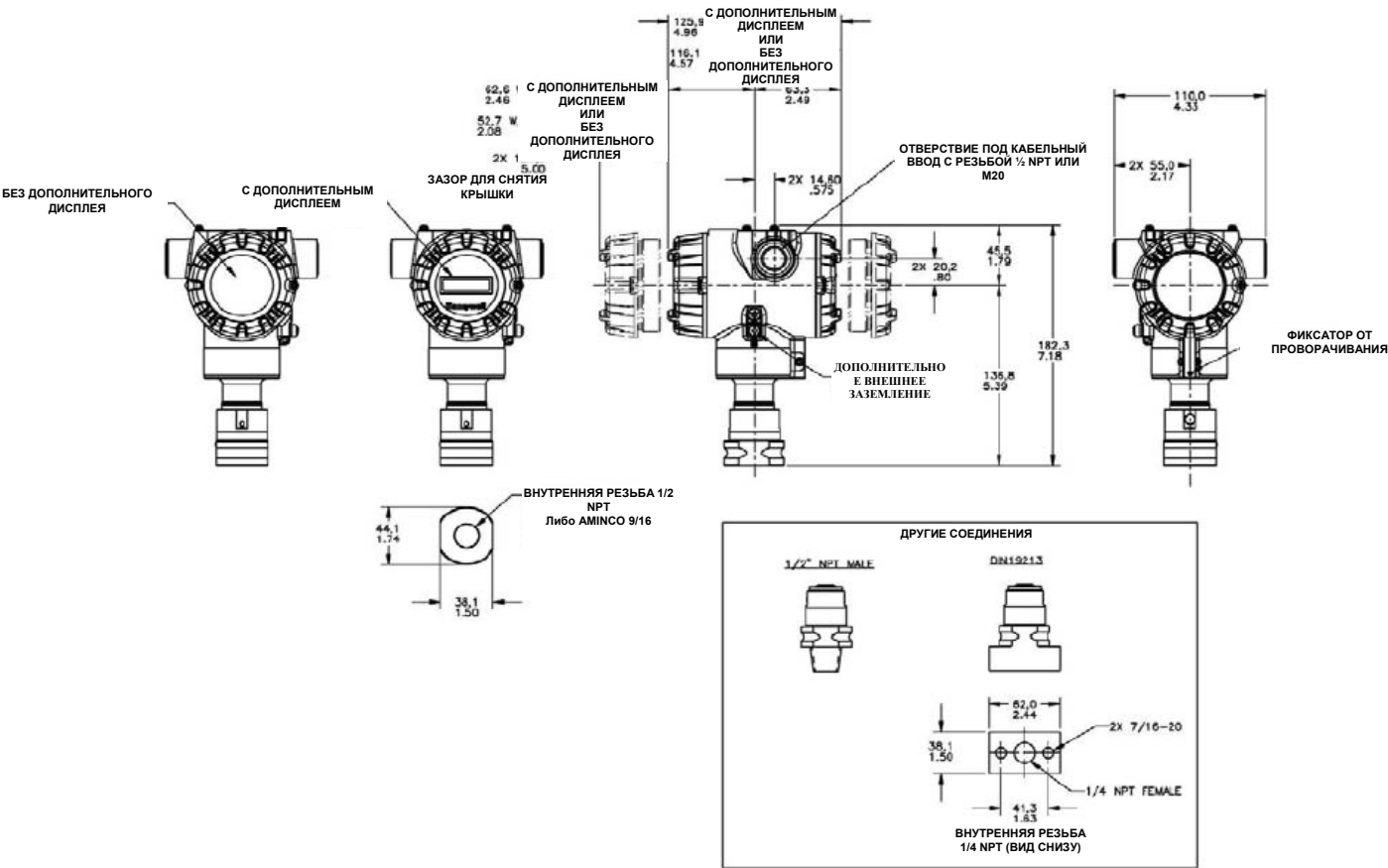
Рисунок 6 – Типовые монтажные размеры STA82L, STA84L и STA87L
