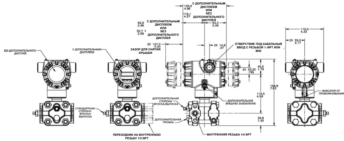
Рисунок 5 – Типовые монтажные размеры STA822 и STA840
